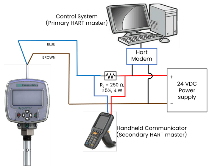
Digitale Kommunikationsverbindungen mit HART-Master-Geräten (Handheld- und Anlagenleitsystem)
