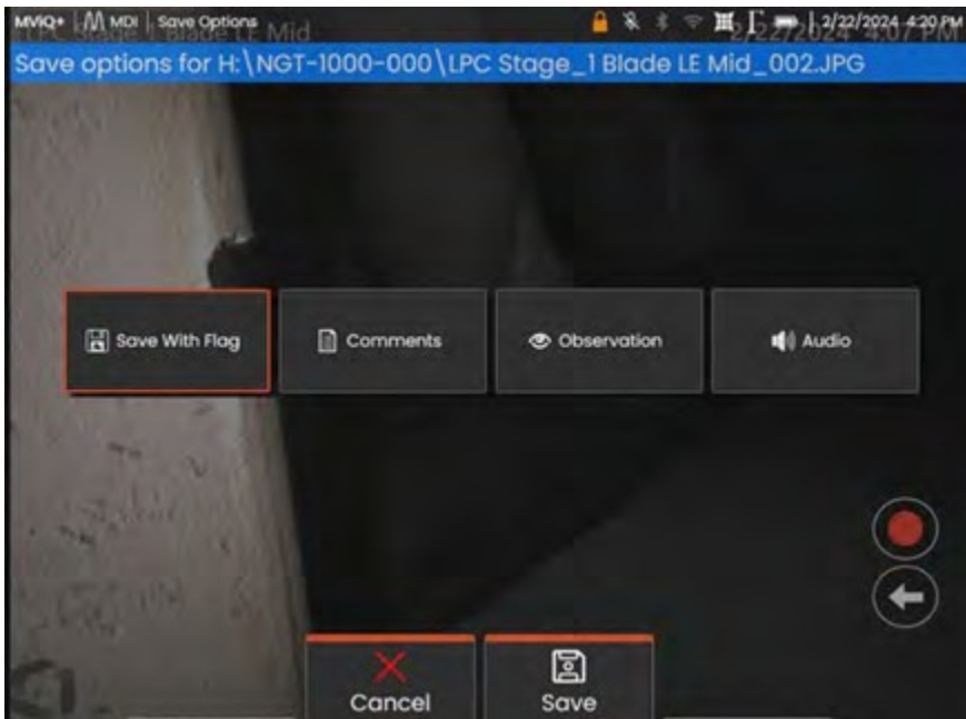
VideoProbe Kommentare & Beobachtungsoptionen vor dem Speichern eines Bildes
