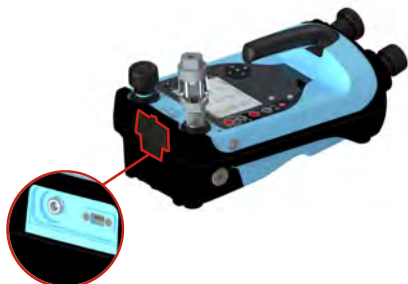
Figur 1: DPI610E laddningsuttag
