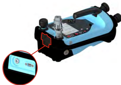
Afbeelding 1: Oplaadpoort DPI610E
