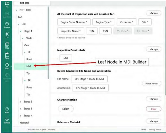
Nodo Hoja en MDI Builder
